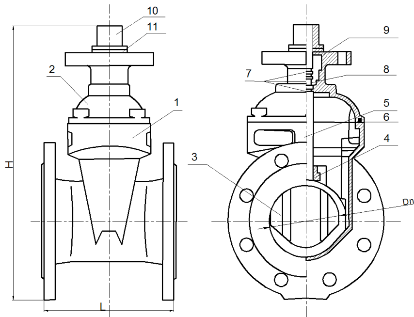
Рис.1 Конструкция задвижки
